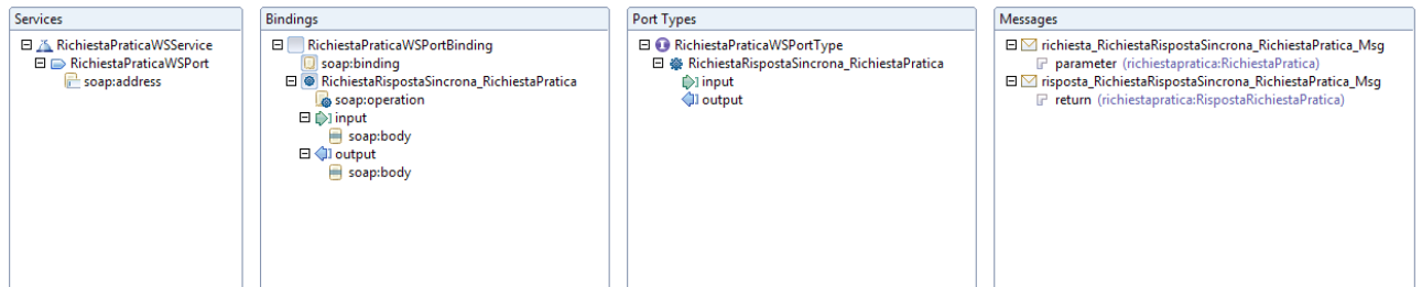
Figura 24. Struttura del WSDL dell'interfaccia RichiestaPratica_WS
